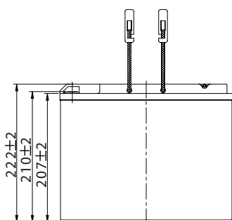
Mått exempel på LPF12-40
